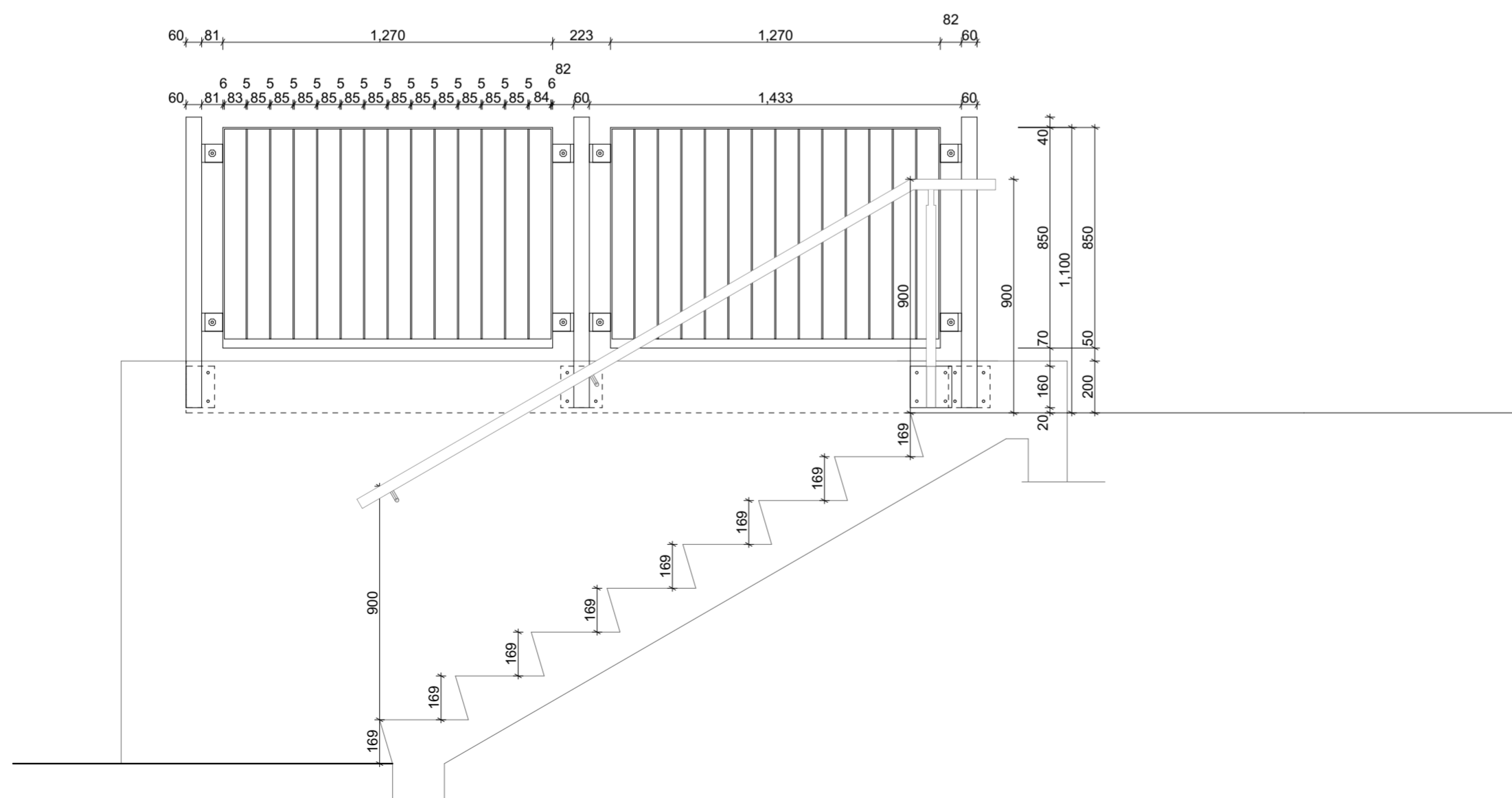
Stigahandrið sneið 1:20
