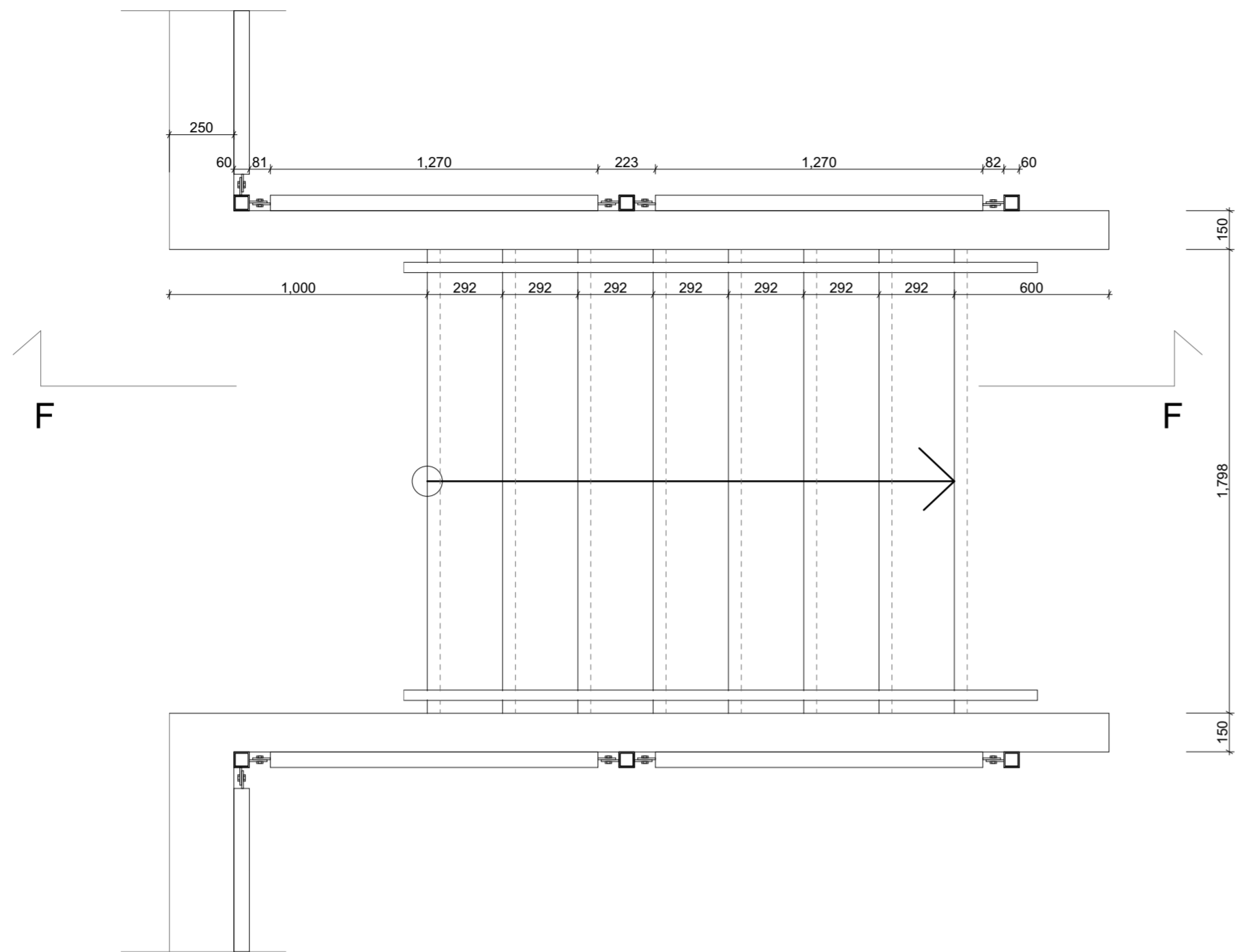
Stigahandrið grunnmynd 1:20
